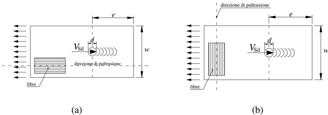
Figura 5-5 – Rifollamento del foro del bullone.
