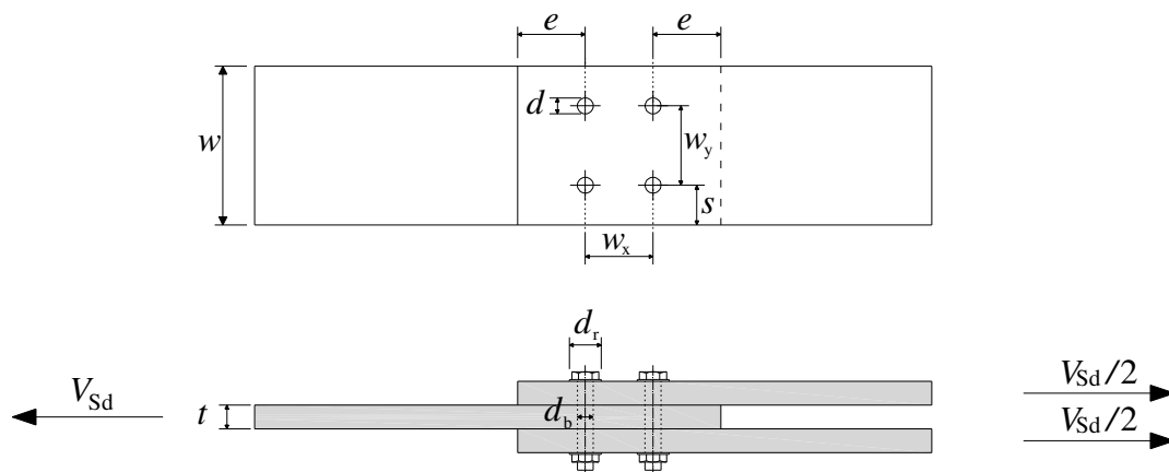
Figura 5-1 – Collegamento bullonato.
