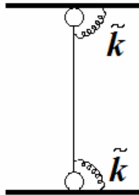
Figura 7-2 – Vincolo offerto dall'anima nei confronti delle ali, che può essere rappresentato tramite molle rotazionali di rigidezza \tilde{k} .
