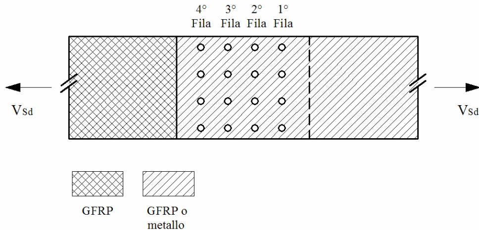
Figura 5-2 – Disposizione delle file dei fori di un collegamento bullonato fra due piastre di FRP o fra un'piastra di FRP ed una in metallo. La risultante delle forze esterne, V_{sd} , è passante per il baricentro della bullonatura.
