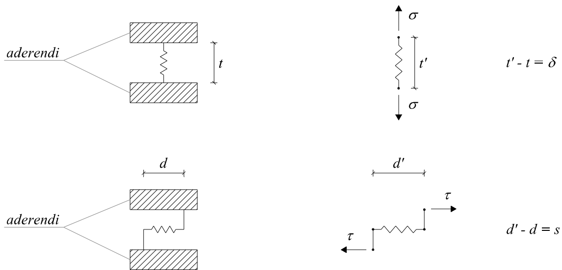
Figura 5-11 – Molle trasversali e longitudinali.
